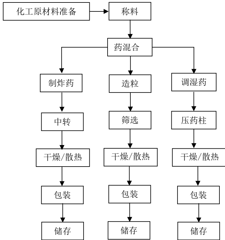
图 2.3-4 炸药、亮珠、药柱生产工艺流程图
