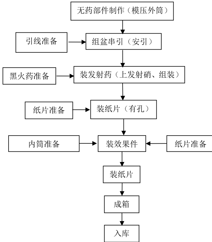
图 2.3-5 组合烟花产品生产工艺流程图
