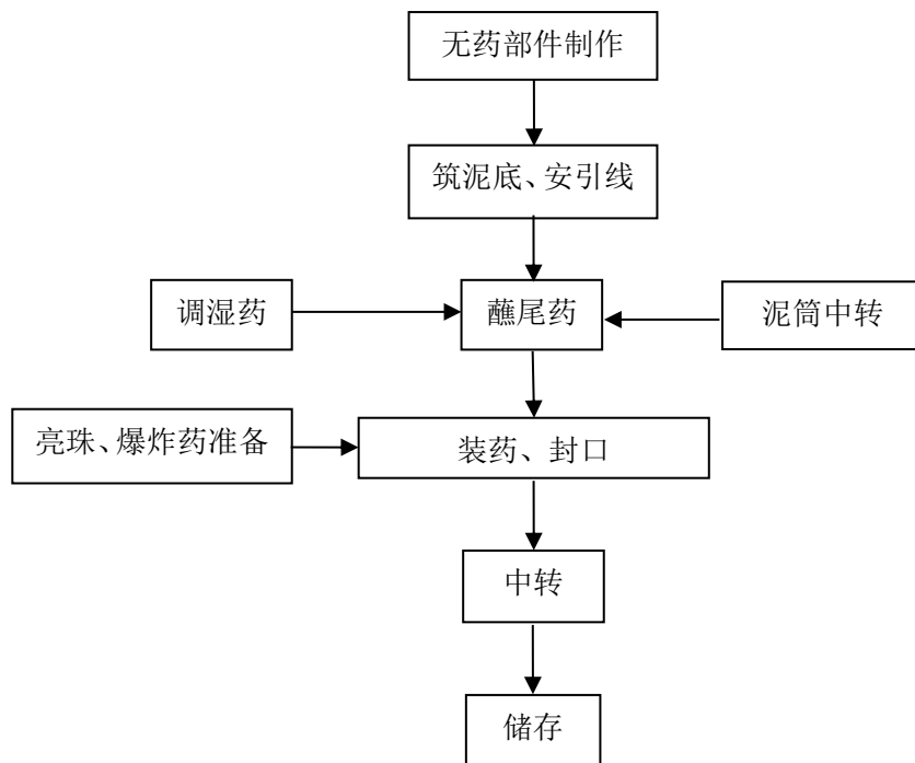
图 2.3-1 效果件内筒（手工装内筒）生产工艺流程图
