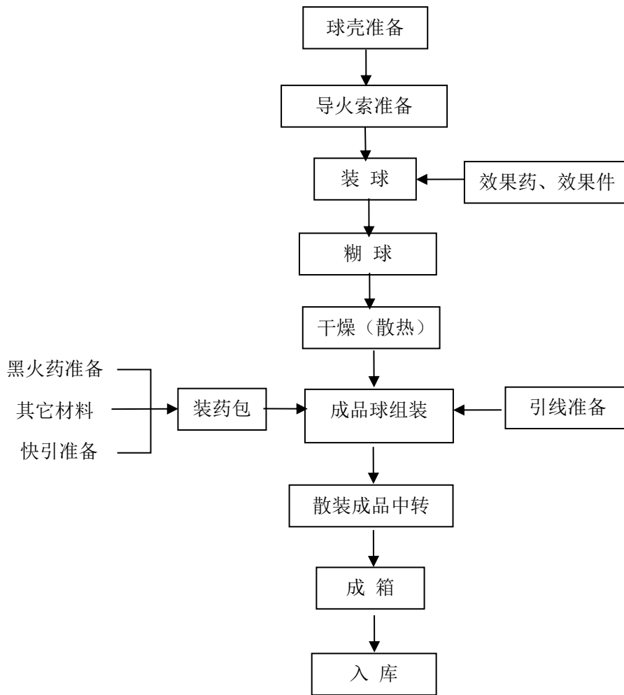
图 2.3-6 礼花类（礼花弹、小礼花）生产工艺流程图
